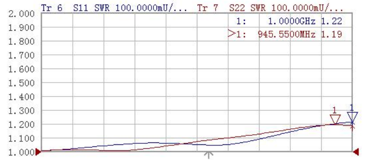
Input/output VSWR
